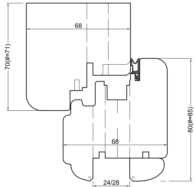
SEZIONE A - A
