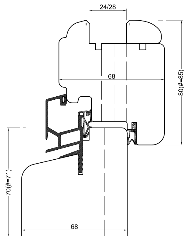
SEZIONE C - C
