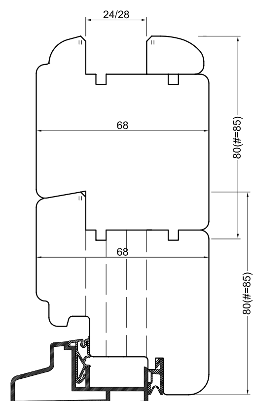
SEZIONE D - D
