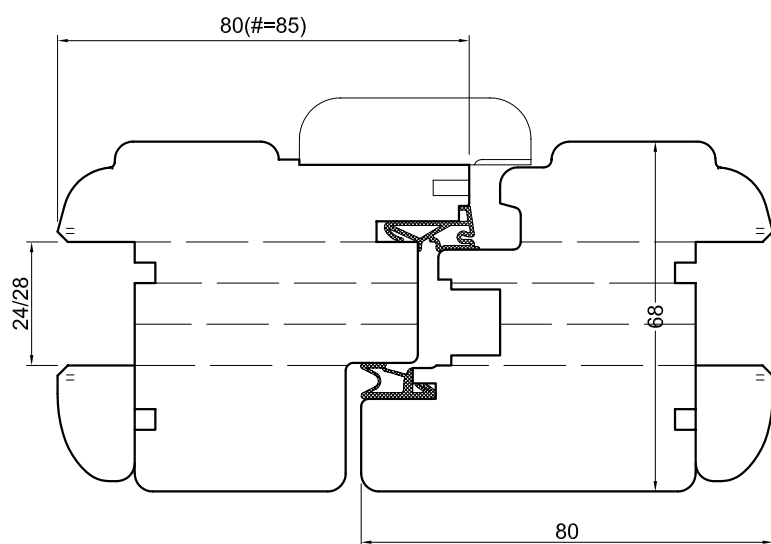
SEZIONE B - B
